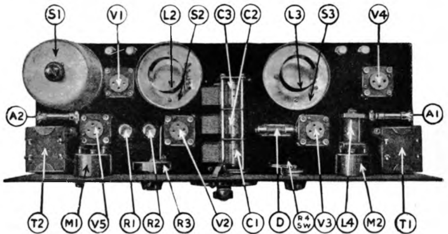
Fig. 5, waarin men de beide h.f. transformators (L2 en L3) herkent. S1 is het schermplaatje van de antenne-spoel, L4 de h.f. smoorspoel, R1 en 2 gloeiweerstanden, A1 en 2 Amperites, M1 en 2 meet-instrumenten, D kristal-detector en R3 volume-regelaar.
